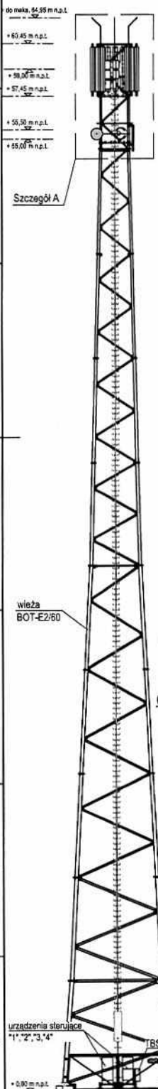
Widok A-A skala 1:200
