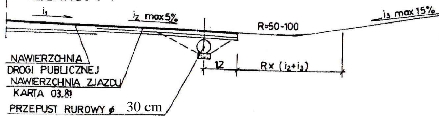
PRZEKRÓJ 1-1
