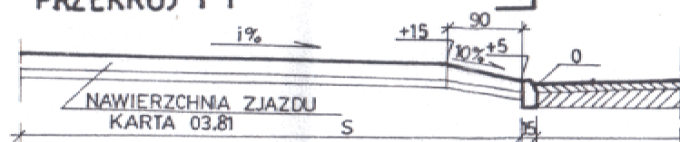
PRZEKRÓJ 1-1
