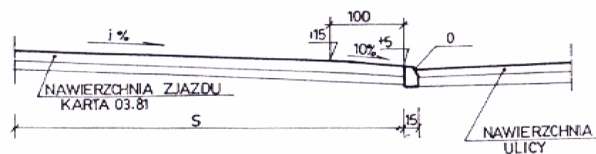
PRZEKRÓJ 1-1
