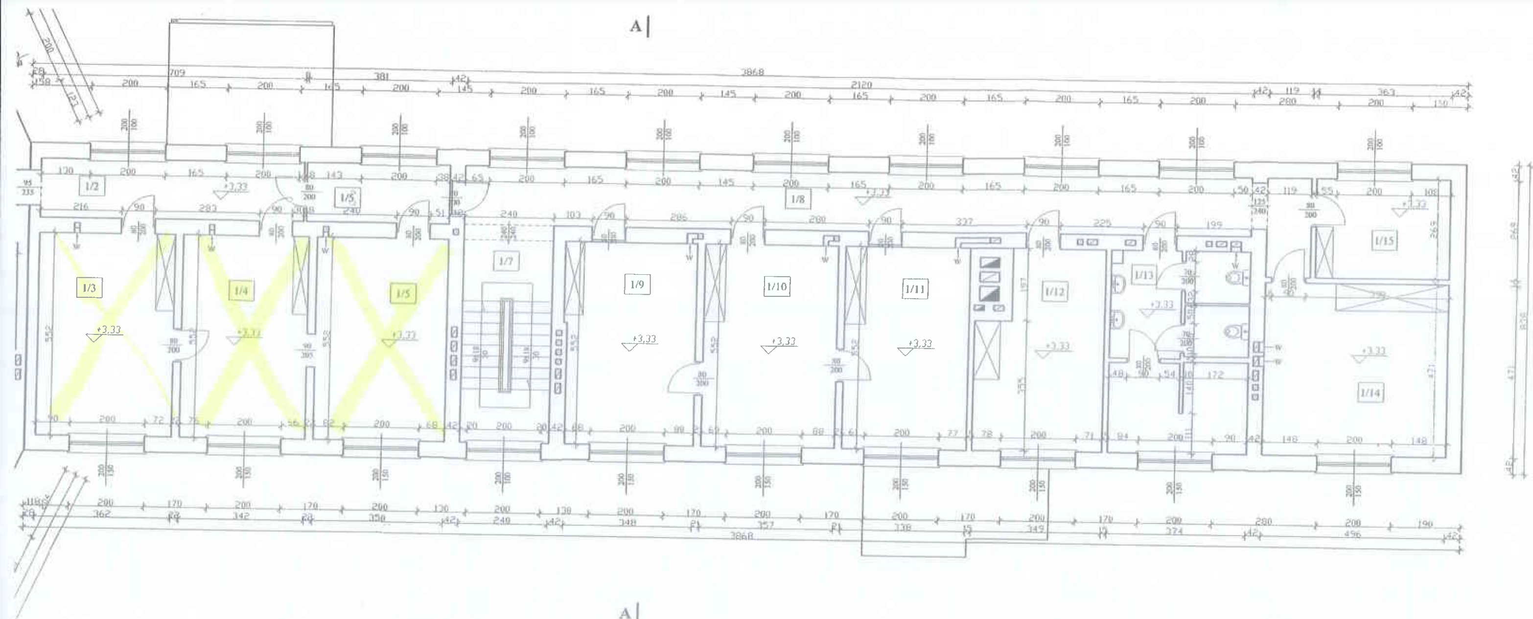
RZUT I PIĘTRA 1:100
